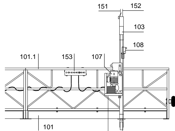
plate-forme avec étriers "C"
