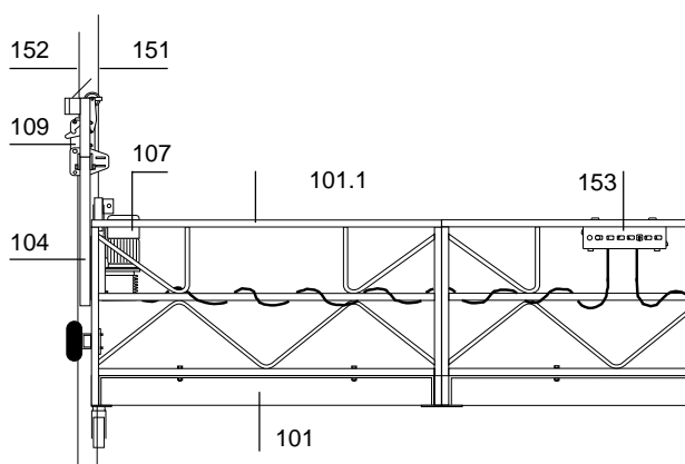
plate-forme avec étriers d'extrémité
