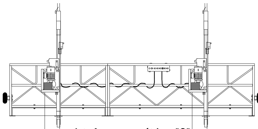
plate-forme avec étriers "C"
